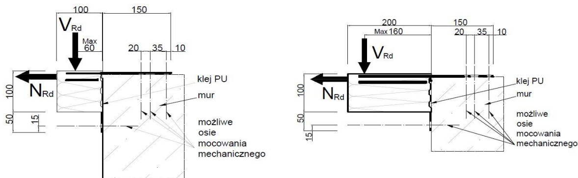
Rys.2. Schematy statyczne elementów CBM zamocowanych w ościeżu (symbole CBM.10.W..... lub CBM.20.W....)
