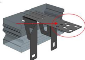
Rys. 1. Schemat usytuowania łączników w zależności od nośności wg tablicy 1
